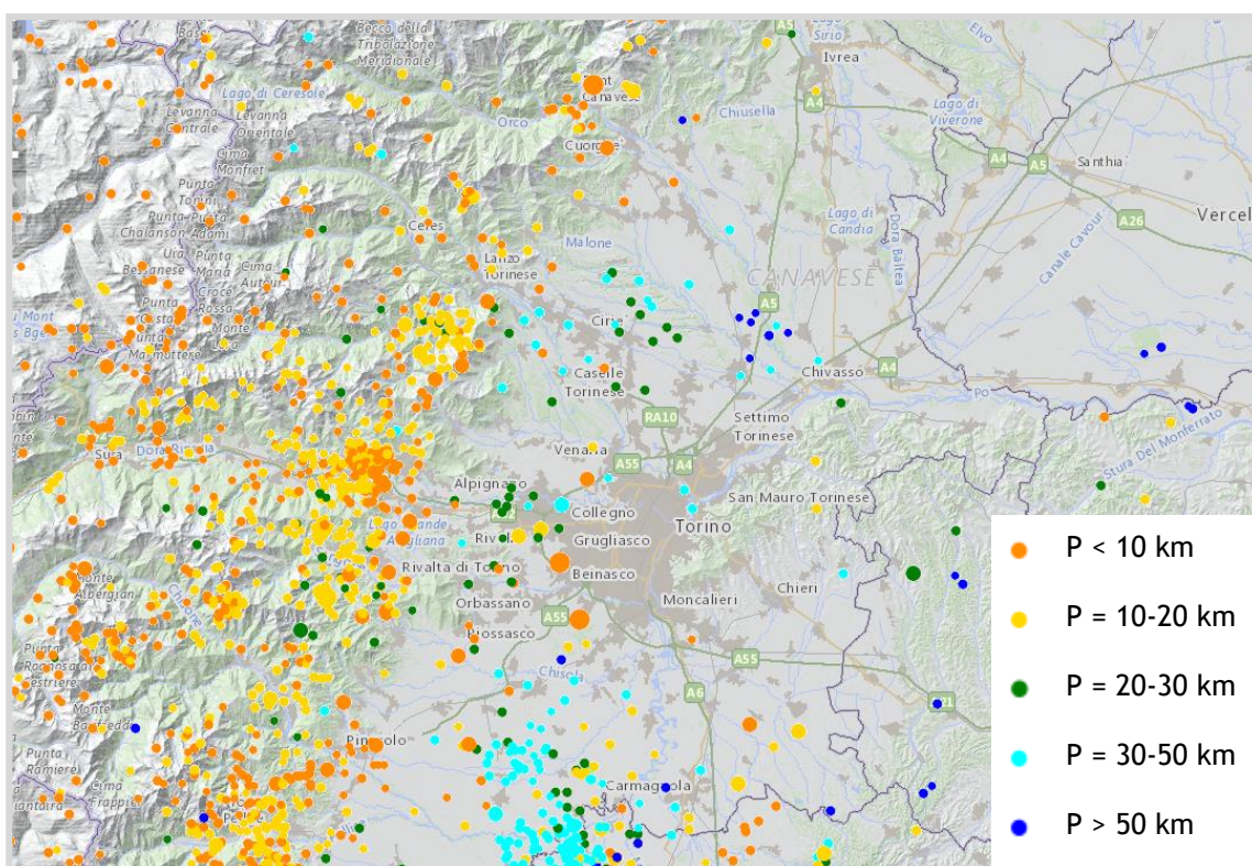
Sismicità storica dal 1982 ad oggi: rappresentazione profondità degli epicentri Regione Piemonte - Arpa Piemonte
